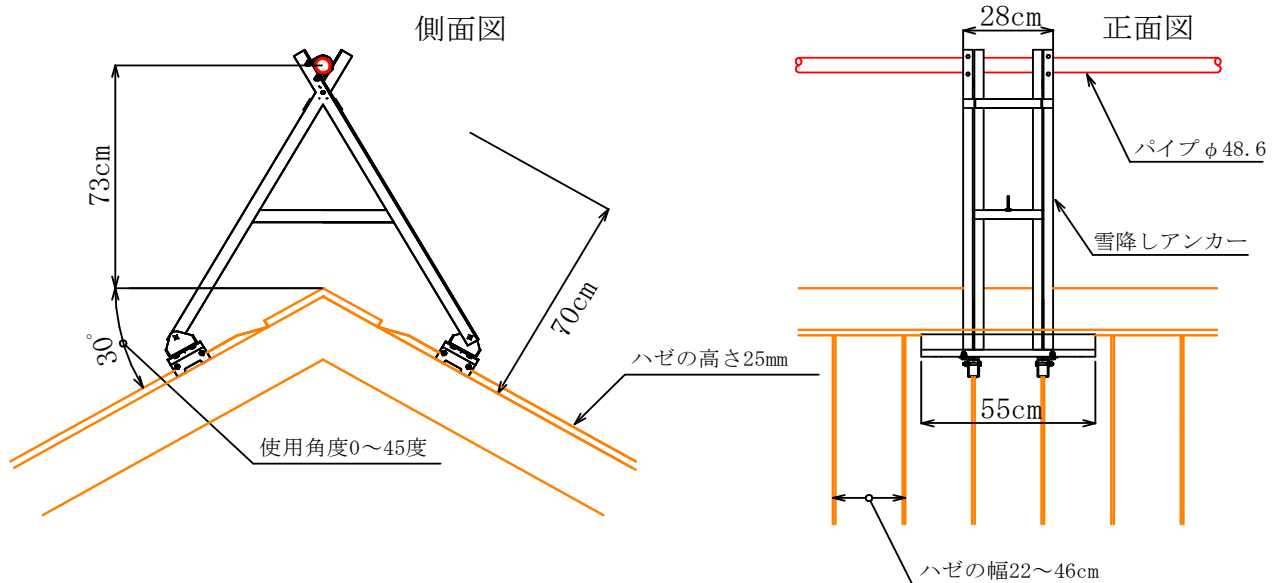
雪下ろしアンカー取付図
